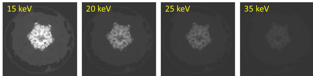
図3 ラット尾の単色 X 線 CT 断面像 (計測像)
