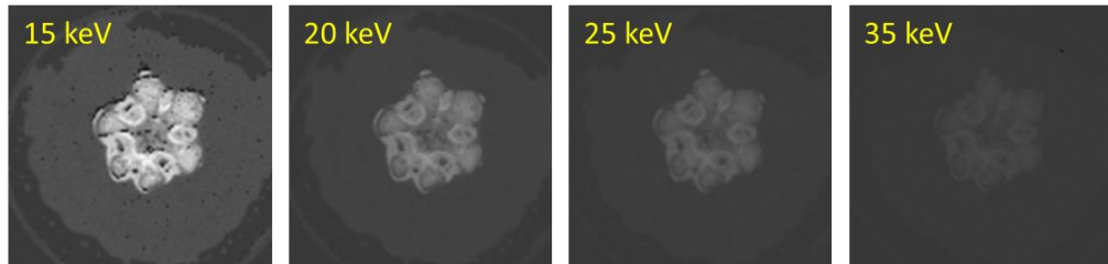
図4 ラット尾の擬単色 X 線 CT 断面像 (計算像)
