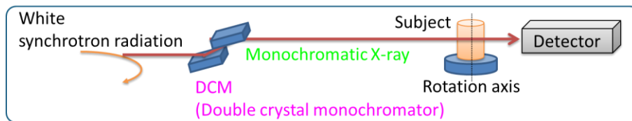
図1 単色X線によるCT計測系
