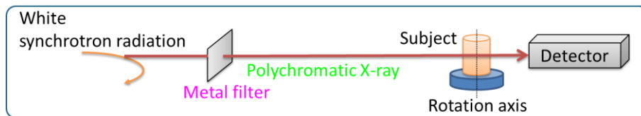
図2 準単色X線によるCT計測系
