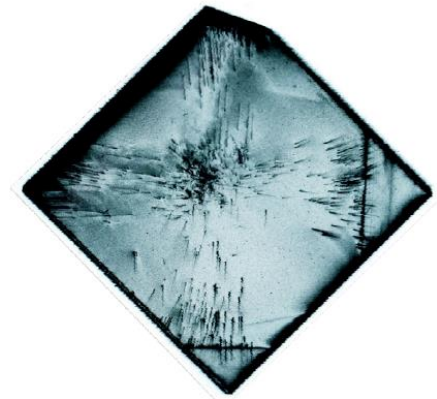
図2 HPHTダイヤモンド（3mm角）のX線トポグラフィ撮影像
