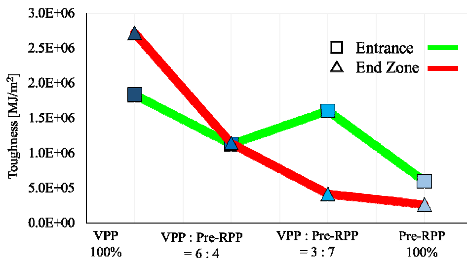
Fig.2 引張試験結果(破断エネルギーまとめ, Entrance:入り口側, End Zone:出口側)
