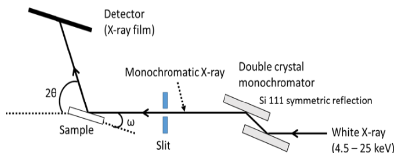
反射配置
