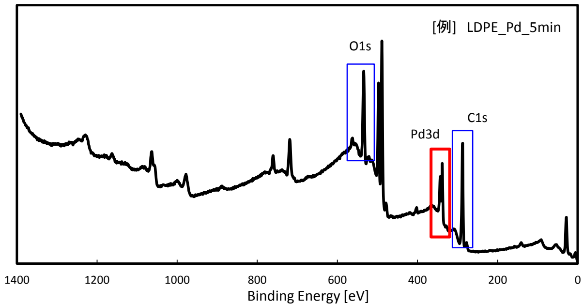
Fig.4 XPS 広域スペクトル (LDPE_Pd_5min).
