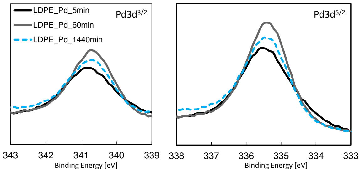
Fig.5 改質時間の違いによる Pd ピークのシフト状態の比較
