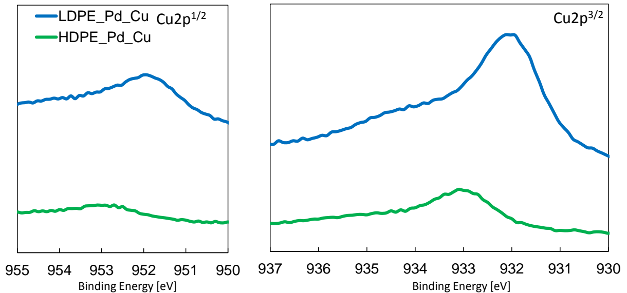
Fig.3 基板の違いによる Cu ピークのシフト状態の比較
