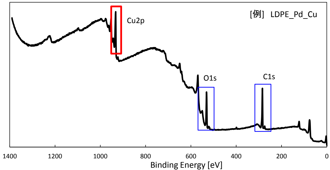
Fig.2 XPS 広域スペクトル (LDPE_Pd_Cu).
