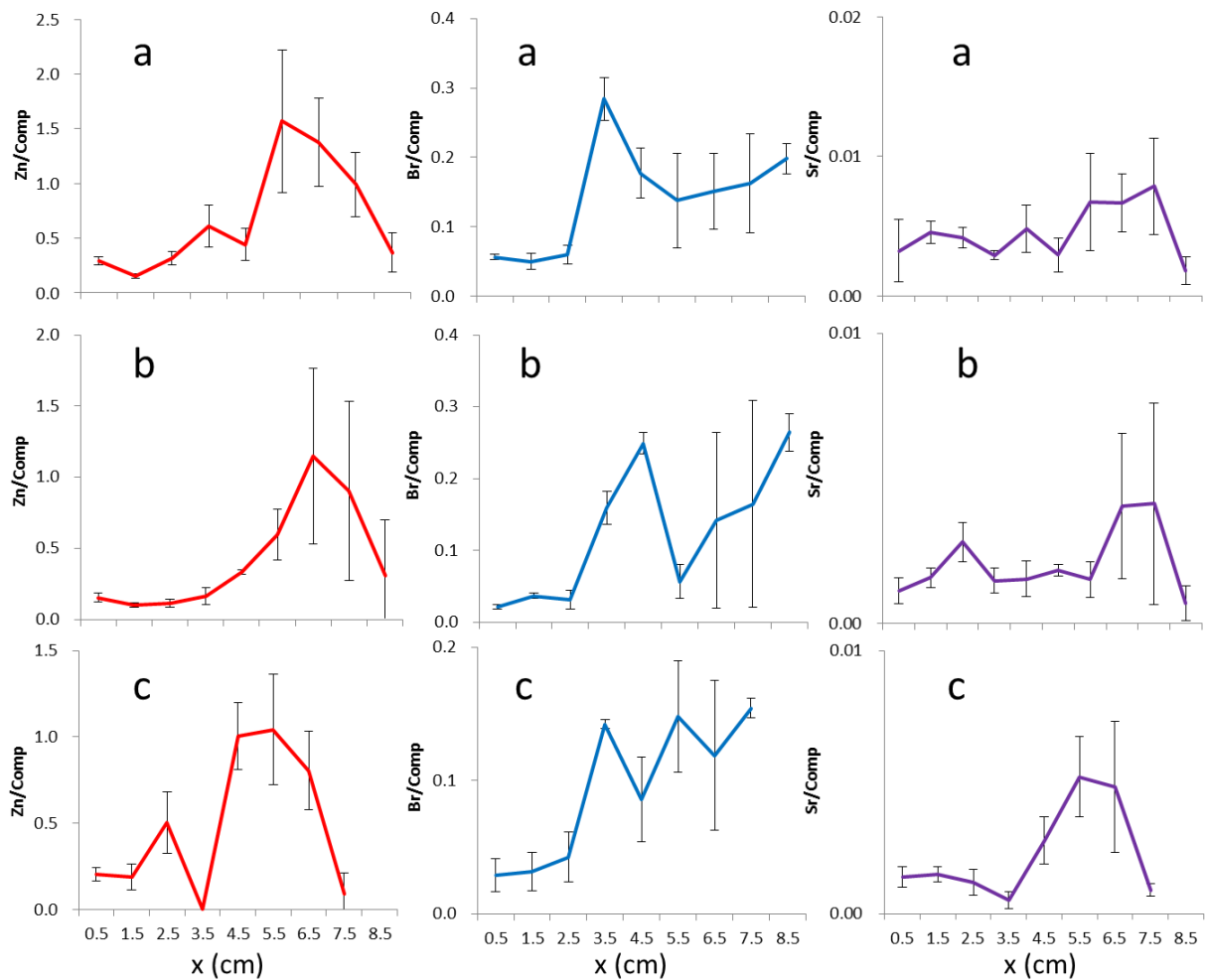
図4 試料 a、b、c における Zn/Comp、Br/Comp、Sr/Comp の分布
