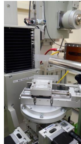
図3 測定のレイアウト
