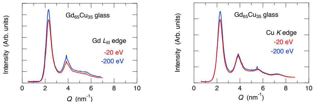
図1：(左) Gd L III および (右) Cu K 吸収端より-20 (赤) および-200 eV (青) で得られた散乱 X 線スペクトル
