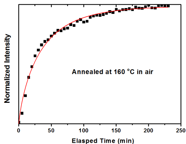
図 3、大気中 160^\circ\text{C} の焼成において、焼成経過時間によりアモルファス \text{In}_2\text{O}_3 薄膜の結晶化度の変化
