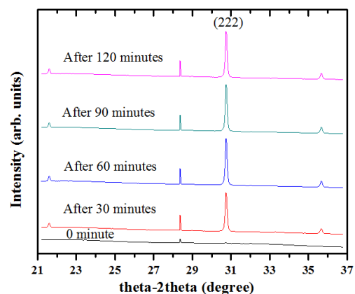
図 2、大気中 160^\circ\text{C} の焼成において、その場 XRD 測定により焼成時間とアモルファス \text{In}_2\text{O}_3 薄膜 (222) 面の増加
